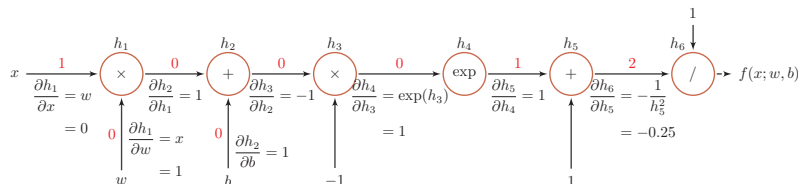
图 4.8 复合函数 f(x; w, b) 的计算图
