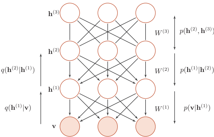
图 12.5 一个有 4 层结构的深度信念网络
