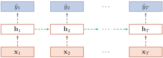
图 7.12 变分丢弃法
