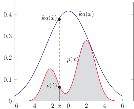
图 11.11 拒绝采样。
