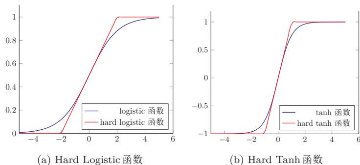
图 4.3 Hard Sigmoid 型激活函数
