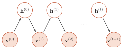
图 12.4 受限玻尔兹曼机的采样过程
