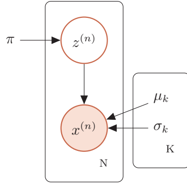
图 11.13 高斯混合模型
