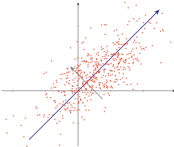
图 9.1 主成分分析
