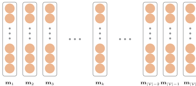
图 15.2 嵌入矩阵
