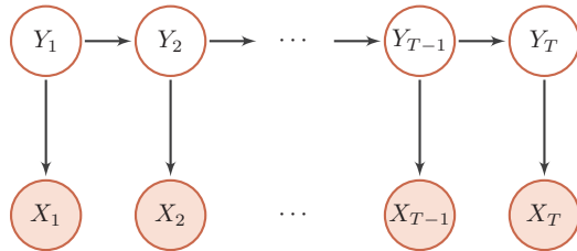
图 11.6 隐马尔可夫模型
